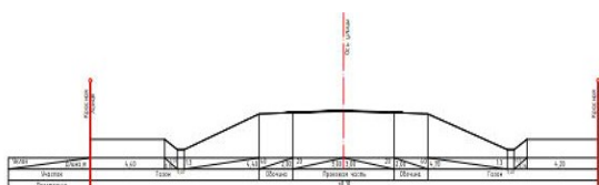
Рис. 4. Поперечный профиль (сечение 1-1)
