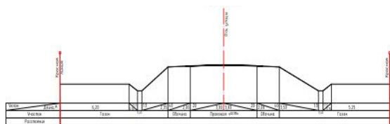
Рис. 5. Поперечный профиль (сечение 2-2)
